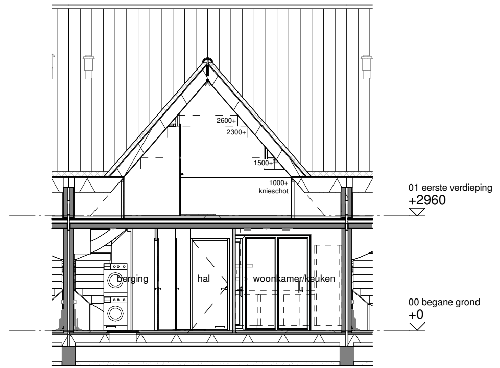
Doorsnede B-B
