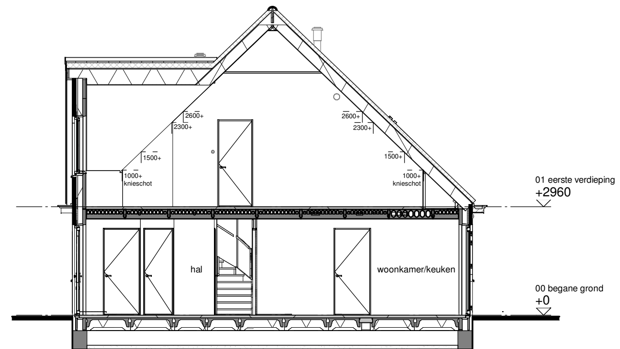
Doorsnede C-C
