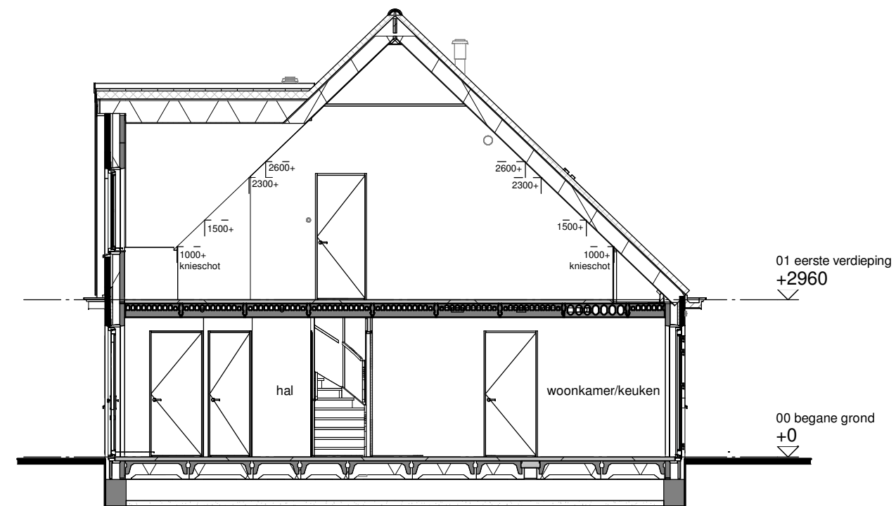
Doorsnede C-C
