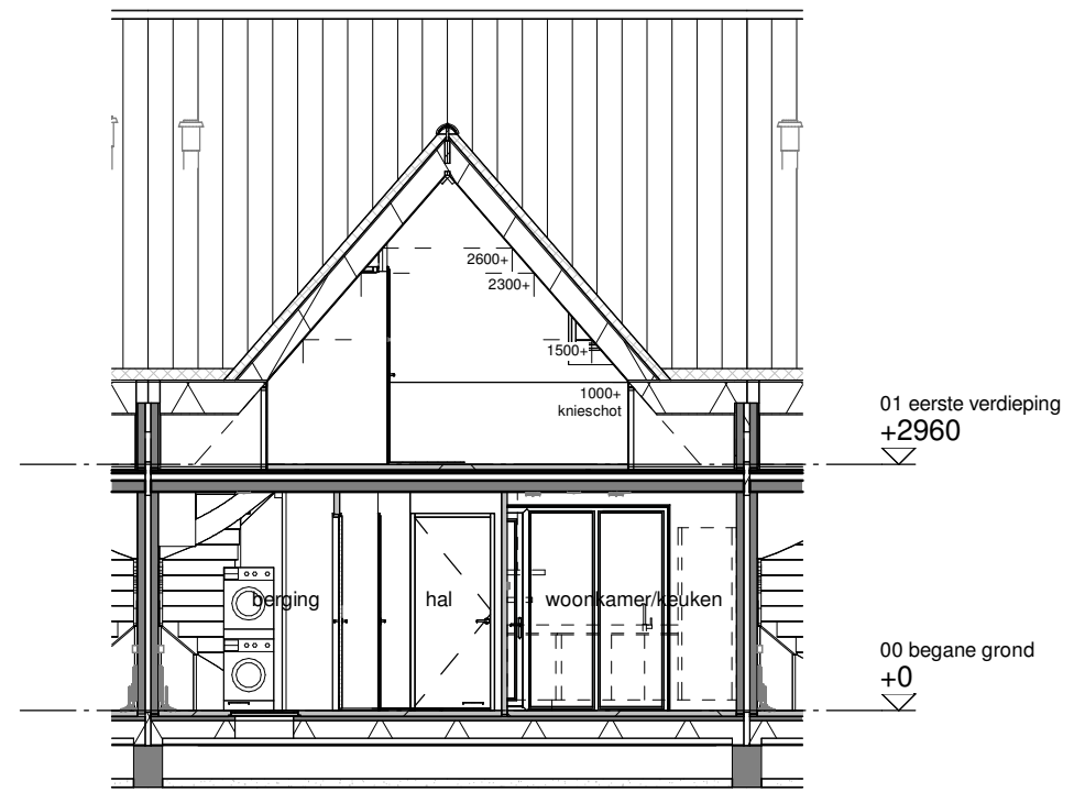
Doorsnede B-B
