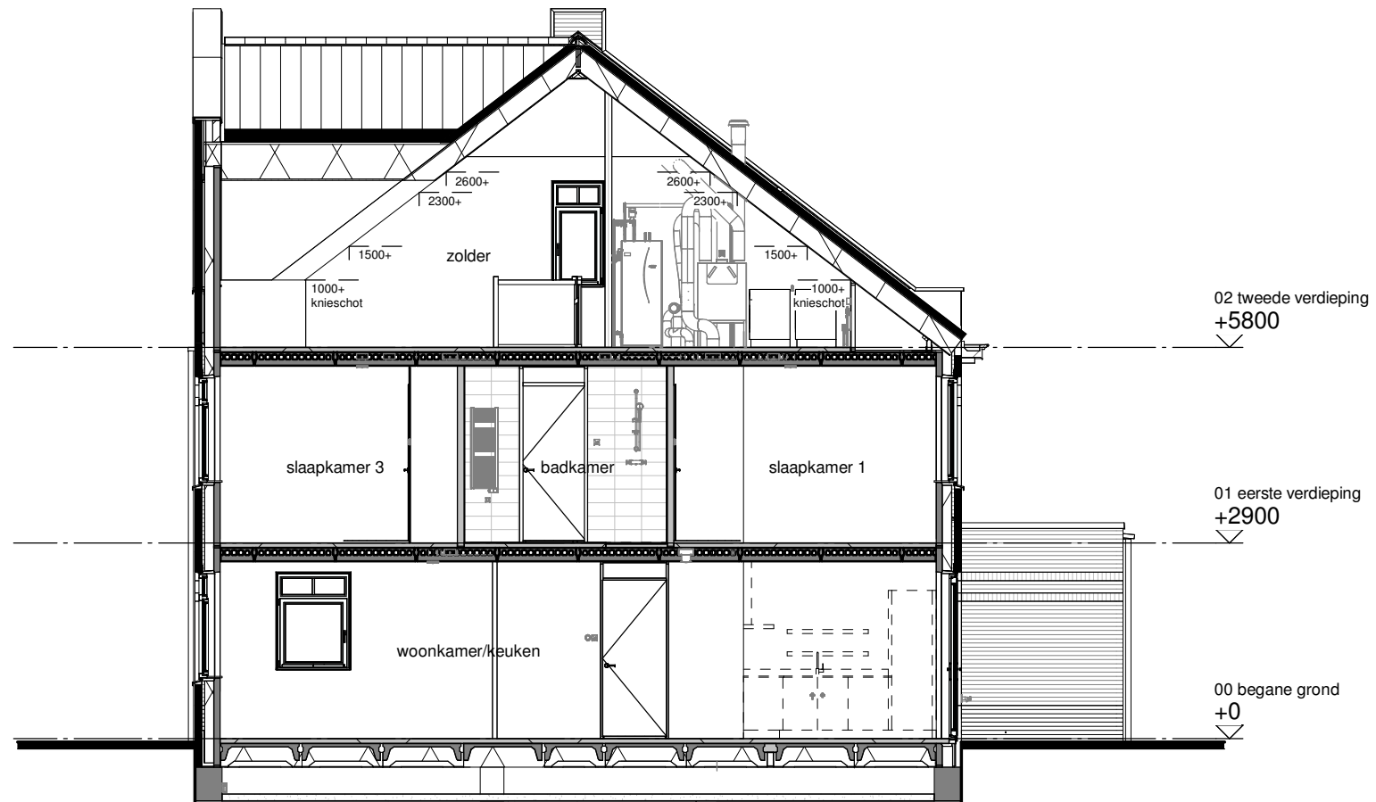
Doorsnede A
