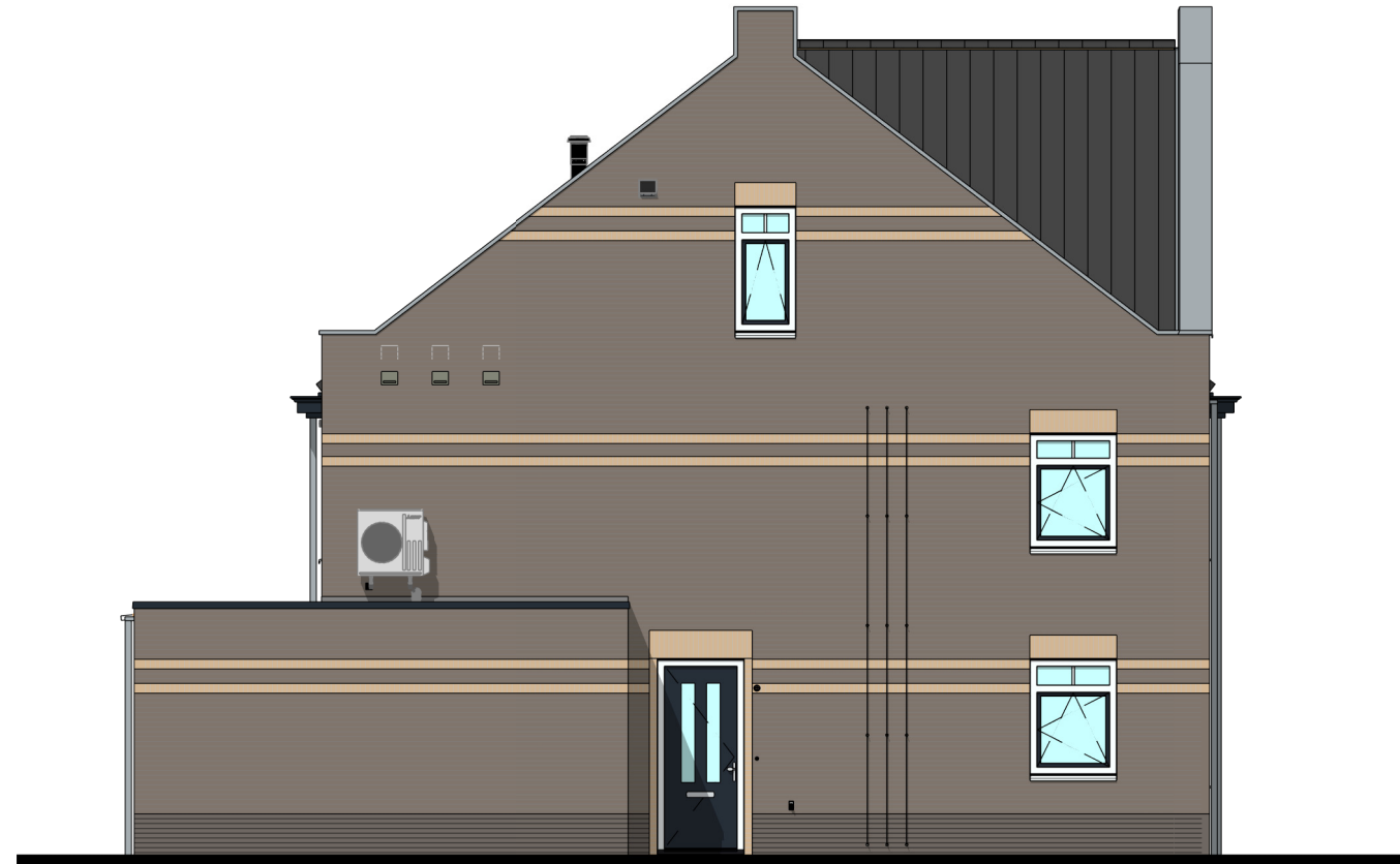
Linker zijgevel
