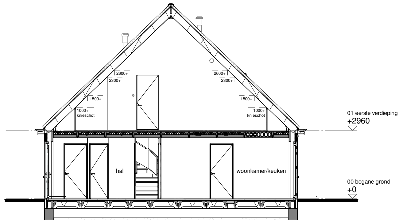
Doorsnede
