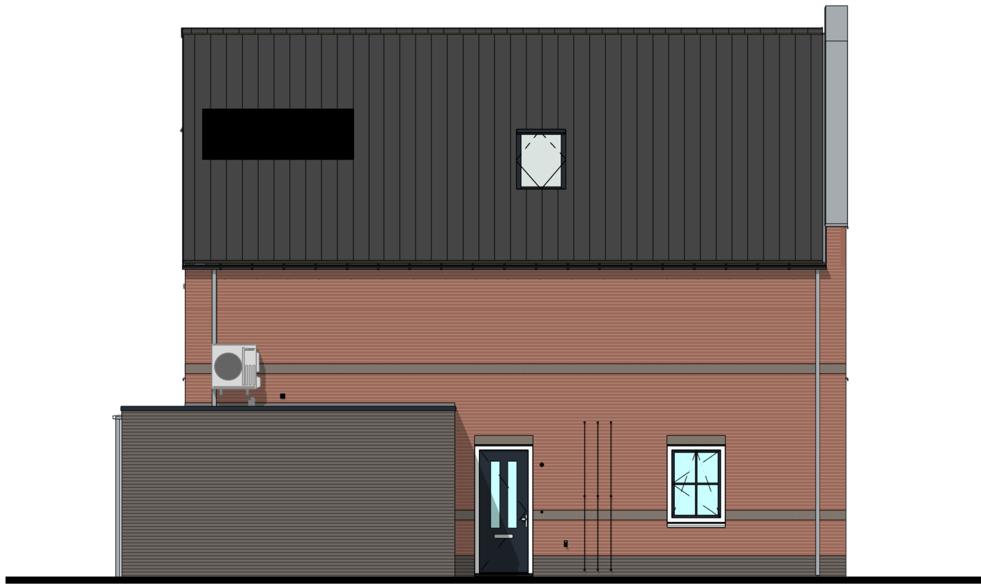
Linker zijgevel
