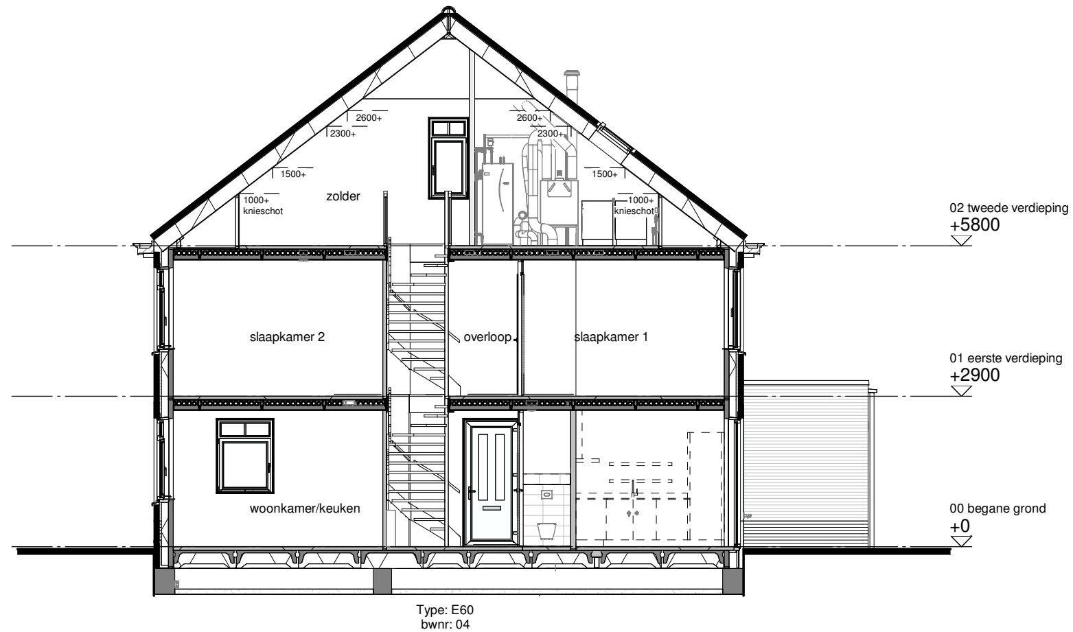
Doorsnede A
