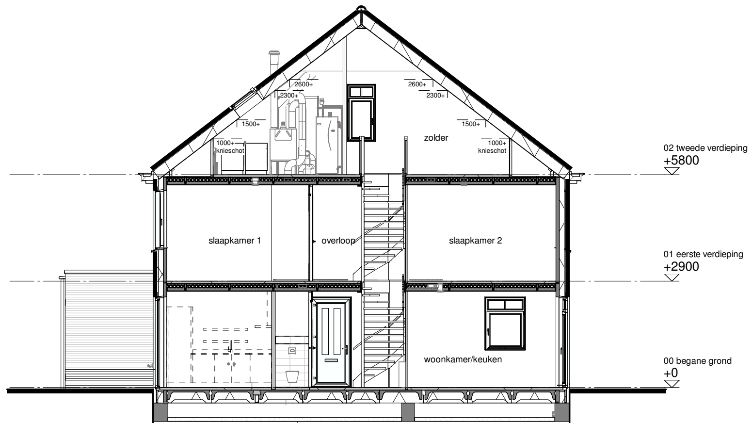
Doorsnede B
