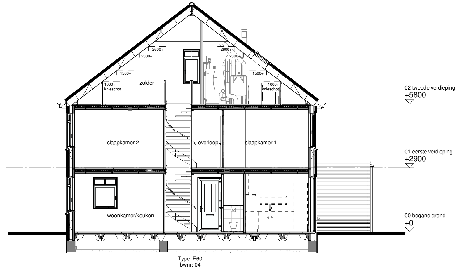
Doorsnede A
