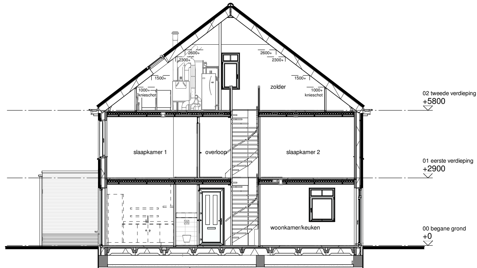
Doorsnede B
